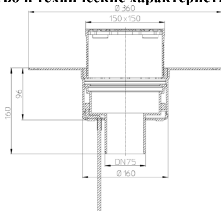
Рис. 1. Кровельная воронка HL62.1BP/7.
