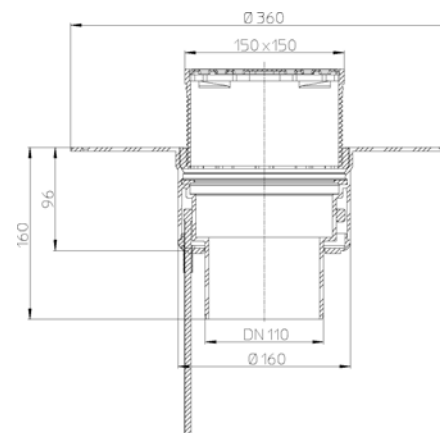
Рис. 2. Кровельная воронка HL62.1BP/1.
