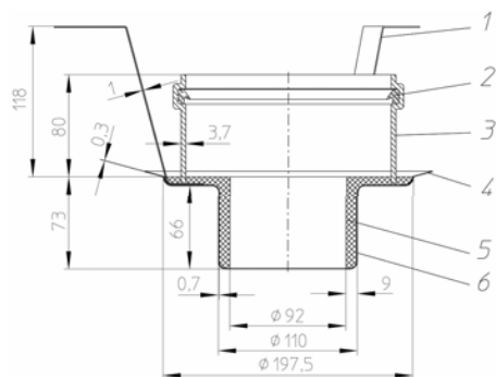
Рис. 6. Противопожарная муфта HL850 для кровельной воронки HL62.1BP/7.
