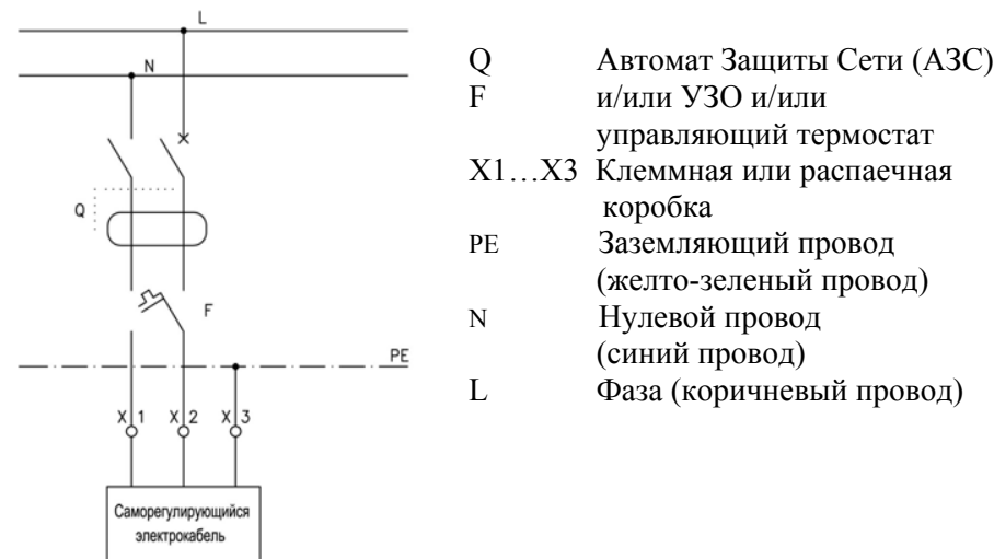
Рис. 5. Схема подключения электрообогрева кровельной воронки HL62.1BP к электрической сети.
