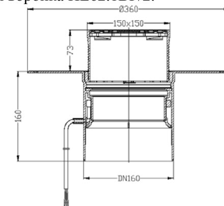
Рис. 4. Кровельная воронка HL62.1BP/5.
