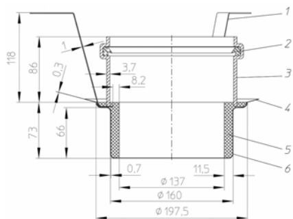
Рис. 7. Противопожарная муфта HL870 для кровельной воронки HL62.1BP/1.
