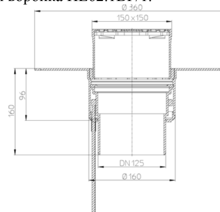
Рис. 3. Кровельная воронка HL62.1BP/2.
